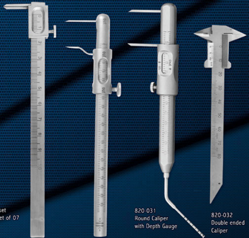
820-029 Sliding Caliper
